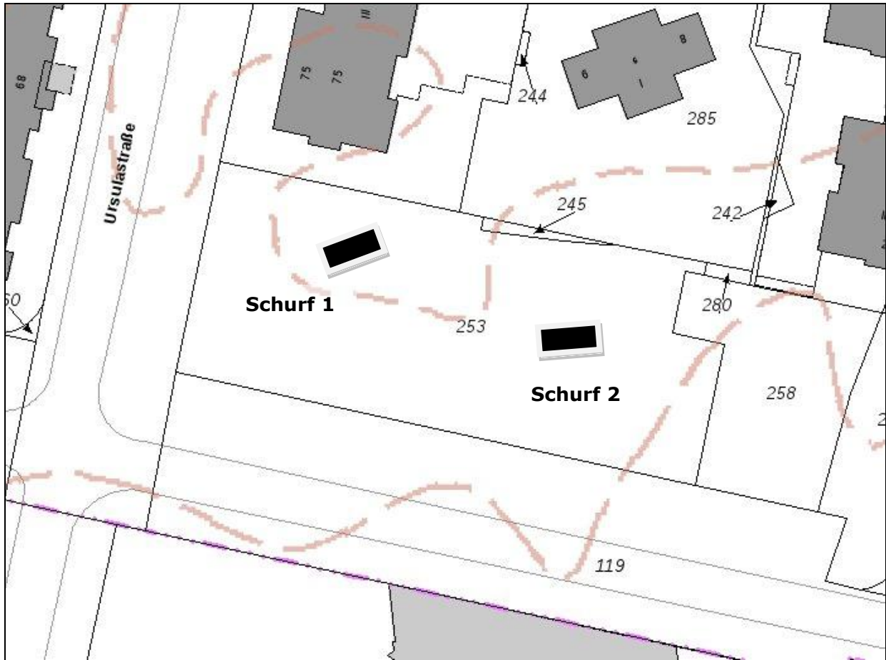
Lageplan Essen Manfredstraße
