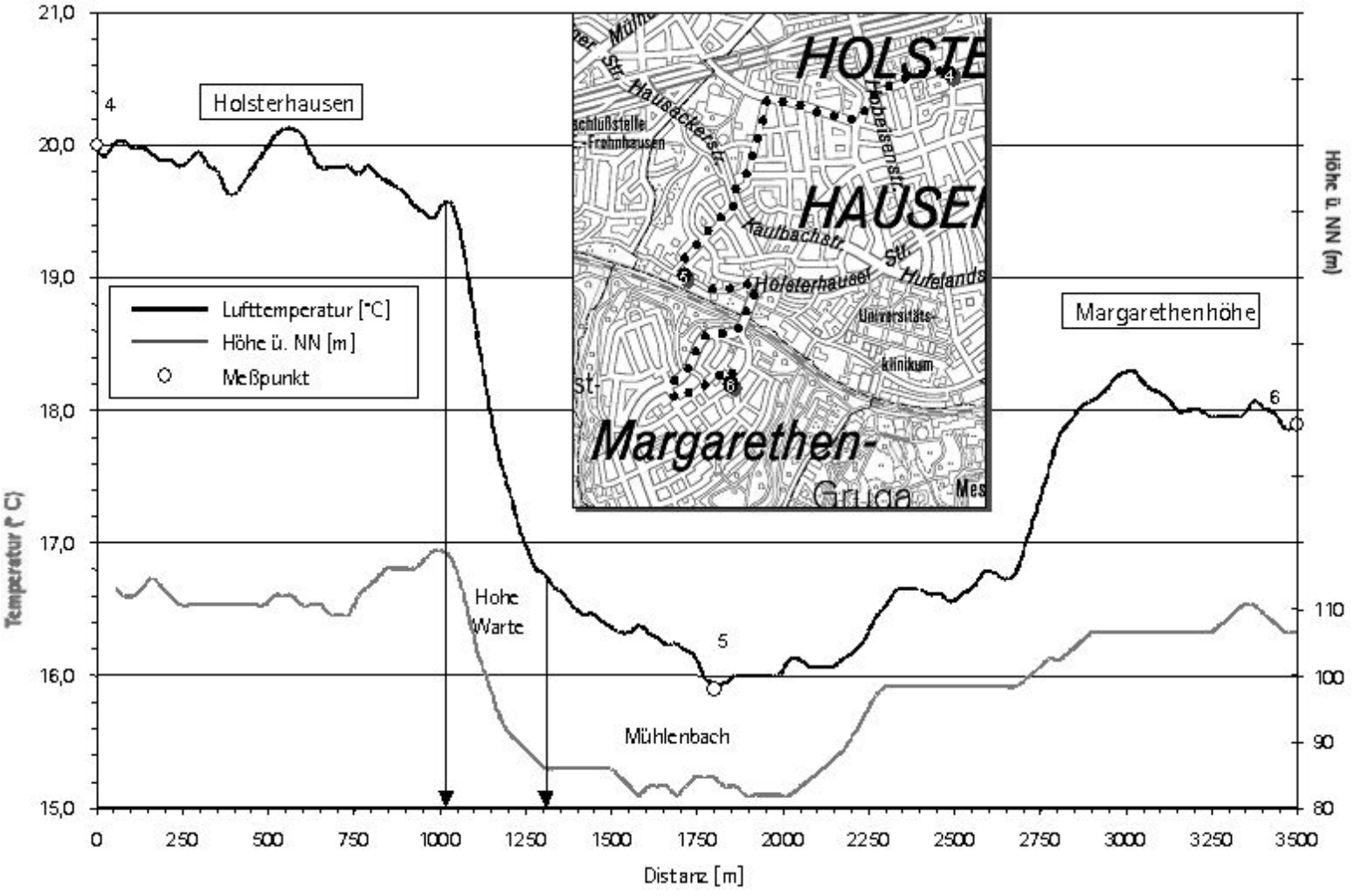
Abb.: Einfluss des Reliefs und der Bebauung auf die Kaltluftdynamik des Borbecker Mühlenbachtals Datengrundlage: 10 Sekundenintervalle der Messfahrt 14 vom 12.08.2000
