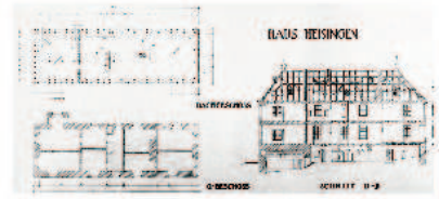
Schnittbild Bauzeichnungen
